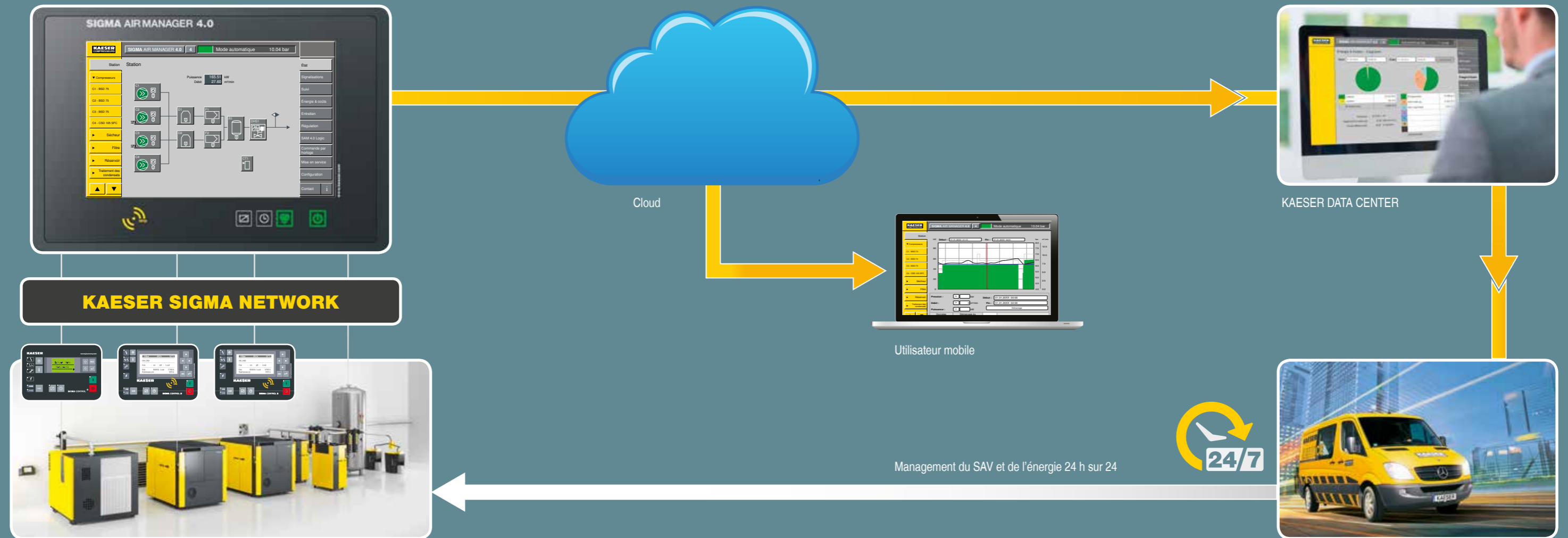
Exemple de station d'air comprimé gérée par le SIGMA AIR MANAGER 4.0
